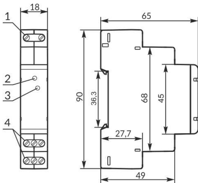
Рисунок 1 – Органы управления, габаритные и установочные размеры ЕМ-130
