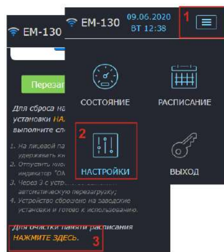
Рисунок 14 – Сброс расписания с Web-интерфейса
