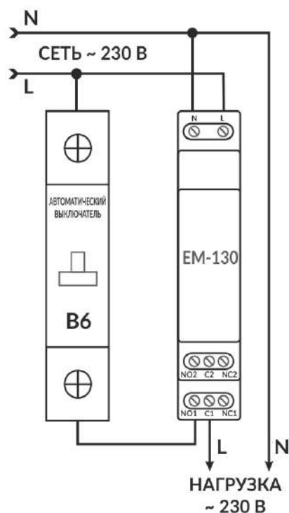
Автоматический выключатель - 6 А класс В
